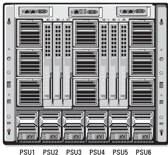
図 8. PSU 6 台構成のシャーシ
